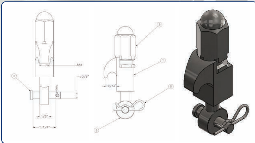
5500 Lid Clamp Assembly
